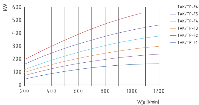
Leistungsdigramm der F-Serie
