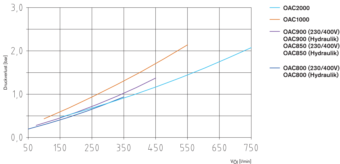
Druckverlustdiagramm
