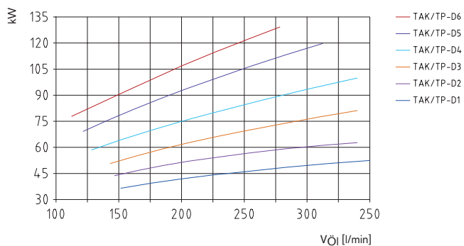
Leistungsdigramm der D-Serie
