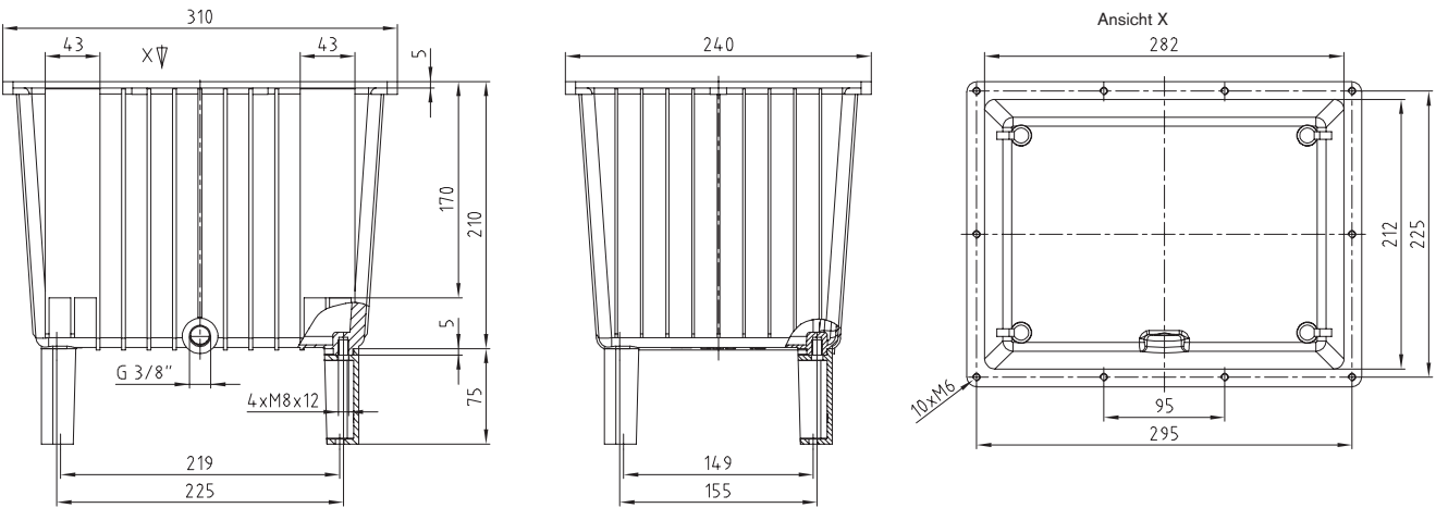
Behälter ohne Ölauffangrand BAK 12
