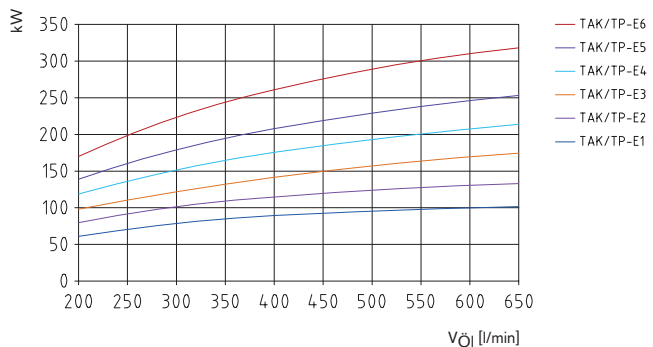
Leistungsdigramm der E-Serie
