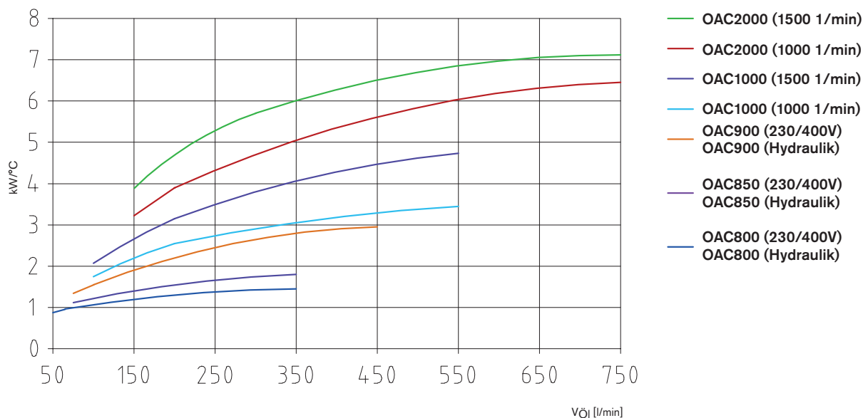
Leistungsdiagramm
