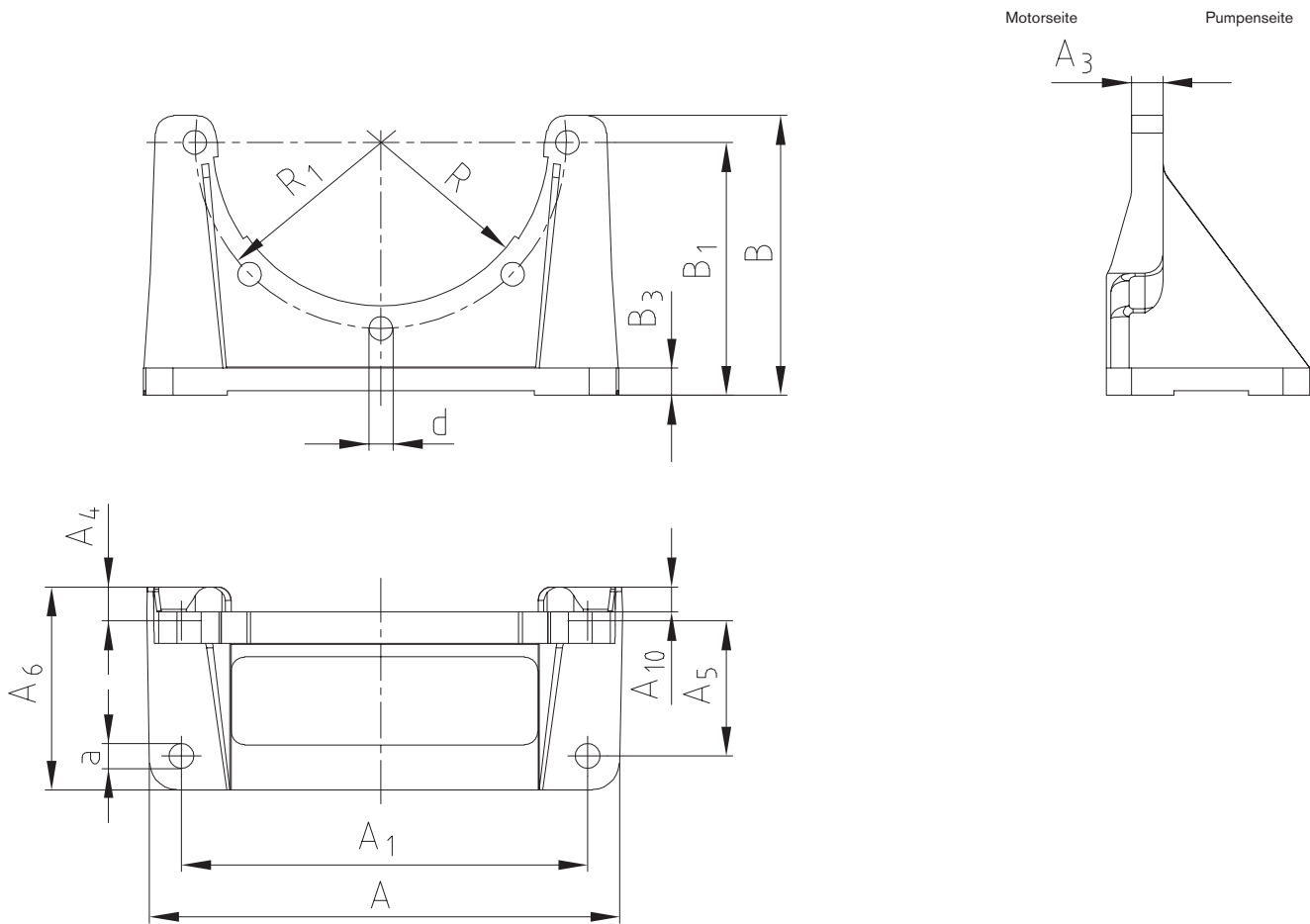
Fußflansch PTFL *
