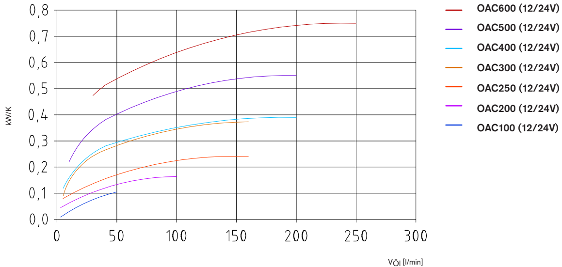
Leistungsdiagramm
