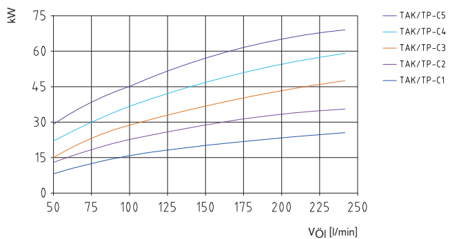
Leistungsdigramm der C-Serie
