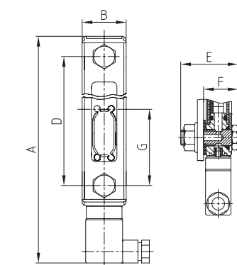
Mit optischer/elektrischer Überwachung des Flüssigkeitsstandes im Behälter KOO/KOS
