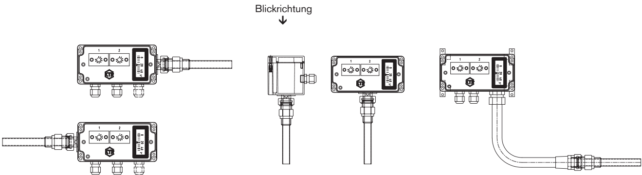
Industrieregler: Bauart/Lage der Tauchhülse
