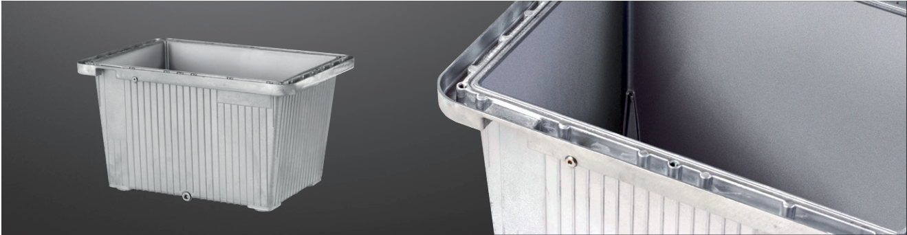
Behälter mit Ölauffangrand BAK 13
