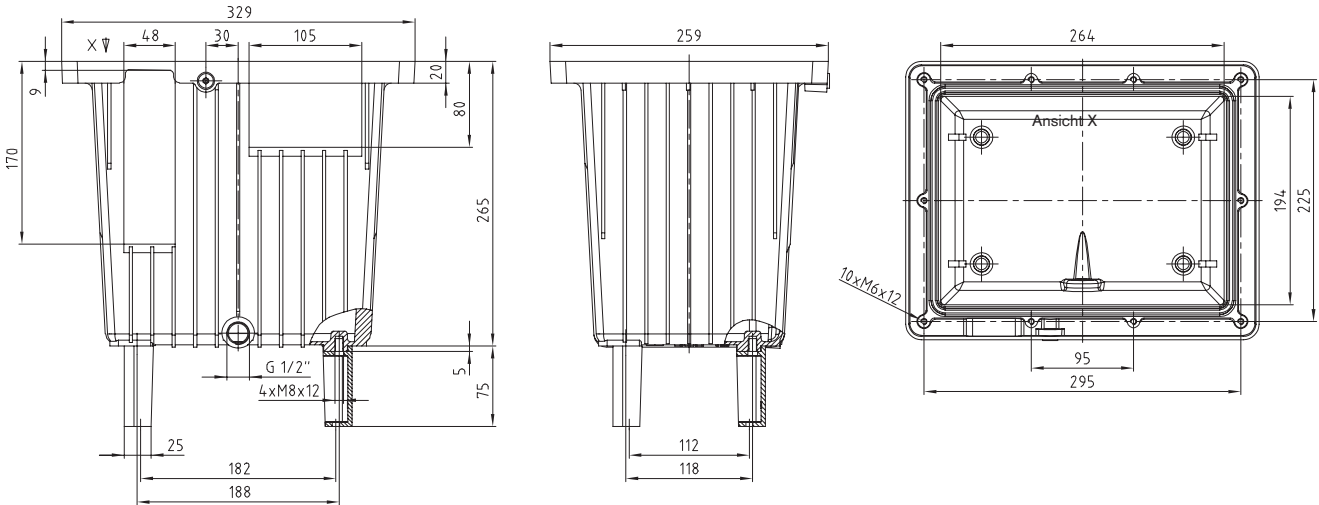
Behälter mit Ölauffangrand BAK 13
