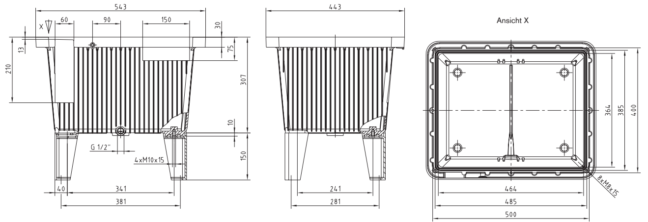
Behälter mit Ölauffangrand BAK 44
