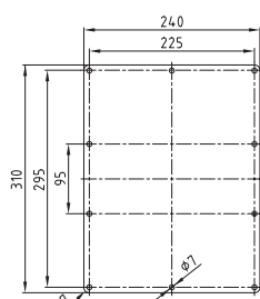
BAK 12 - ST 12 / AL 12 St: 3 mm stark; 1,7 kg
