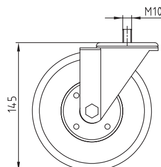
Lenkrollen LR 150 und LR 150 F mit Feststeller
