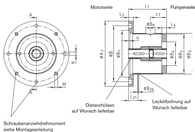
Pumpenträgergröße 350 - 660
