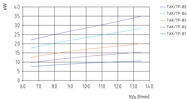
Leistungsdigramm der B-Serie
