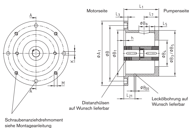
Pumpenträgergröße 160 - 300
