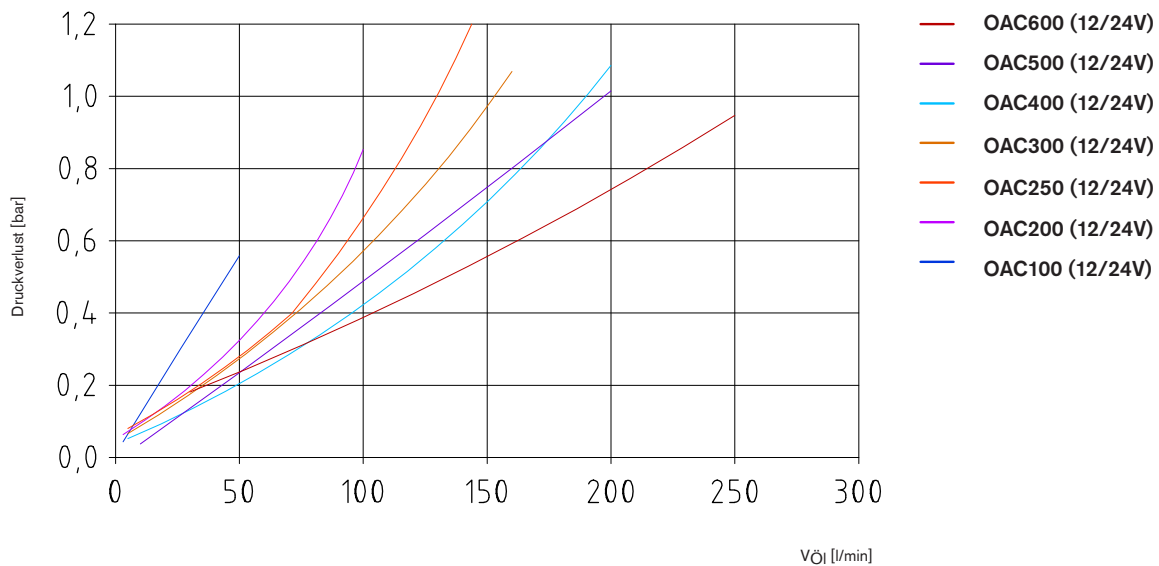
Druckverlustdiagramm
