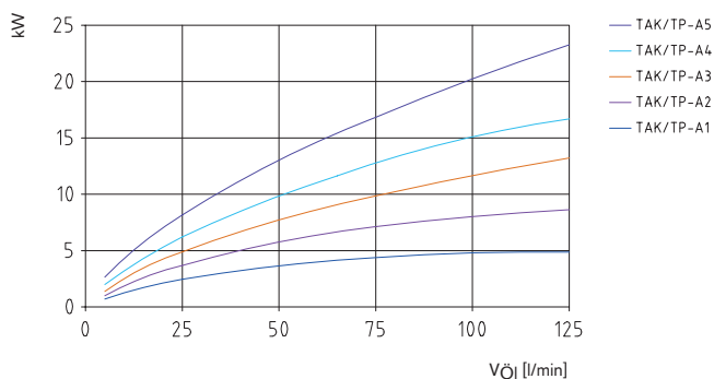
Leistungsdigramm der A-Serie
