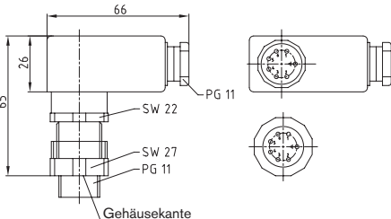
Stecker A03 DIN 43651
