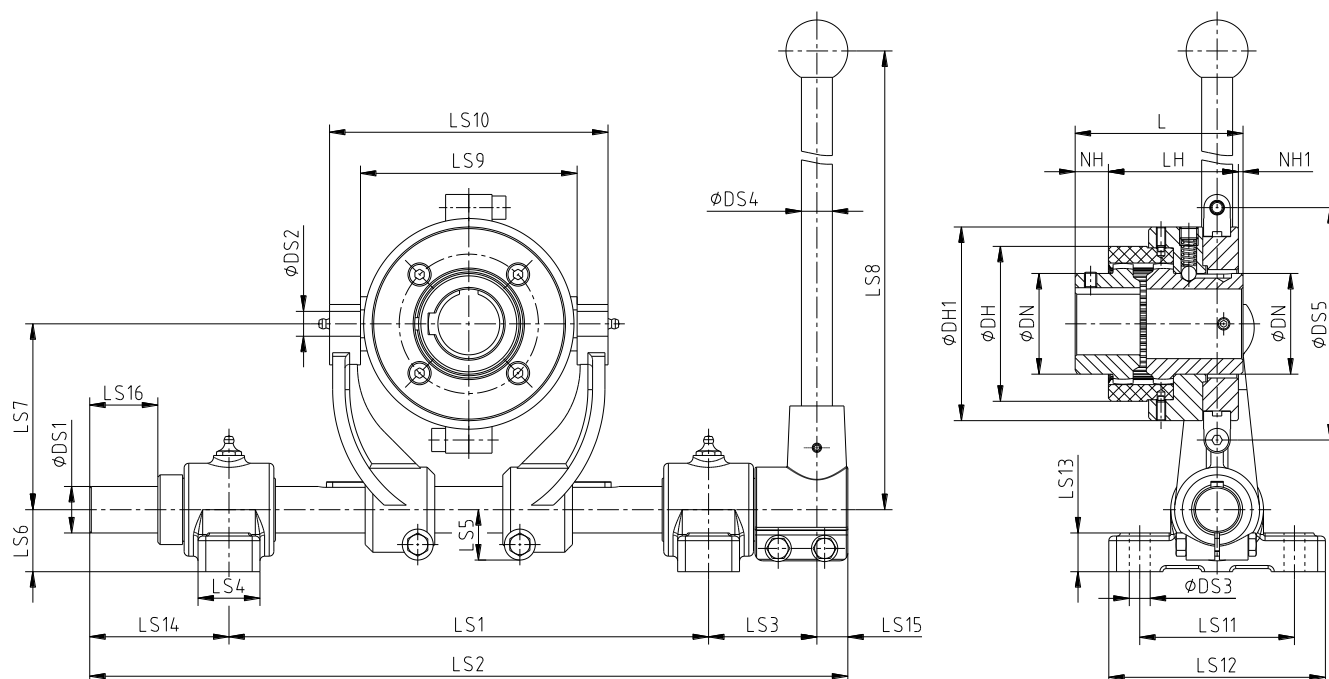
rysunek 3: BoWex® SD1 z mechanizmem przełączającym
