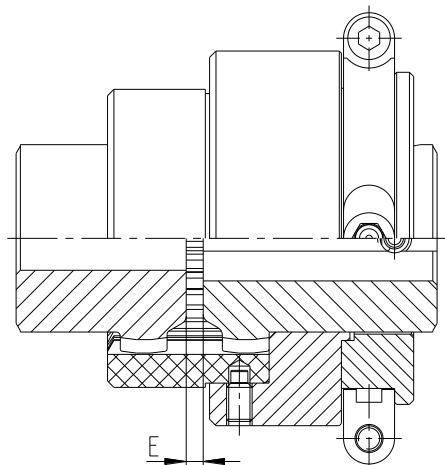
rysunek 15: montaż sprzęgła
